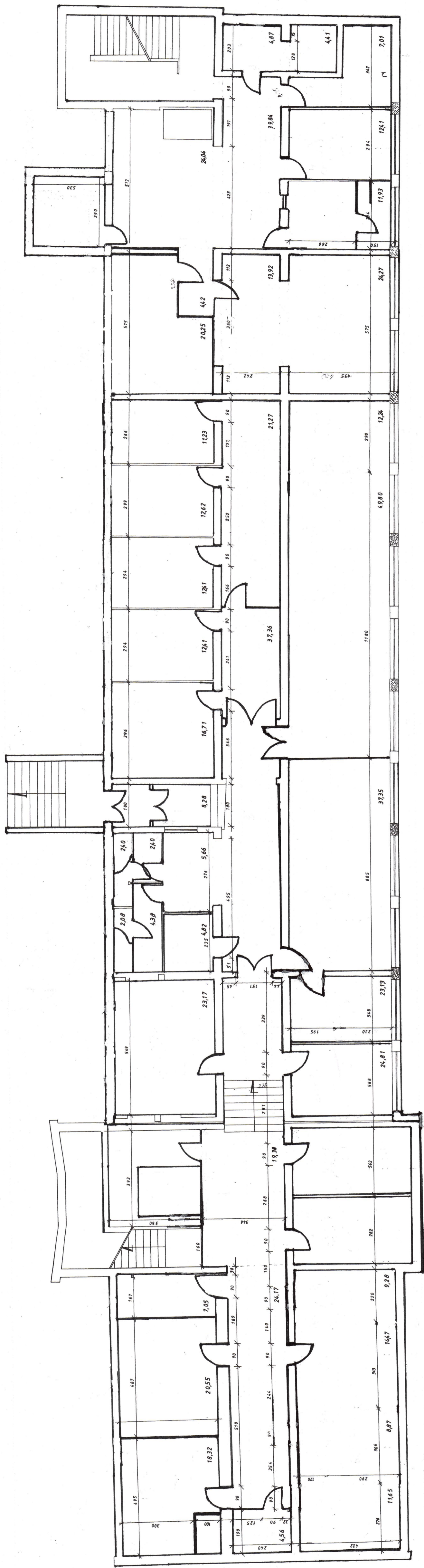
RZUT PIWNIC 1:50
