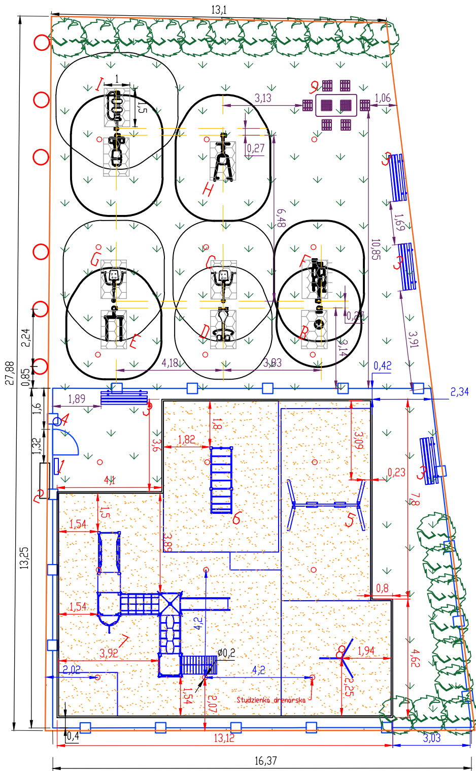
Układ studzienek drenarskich
