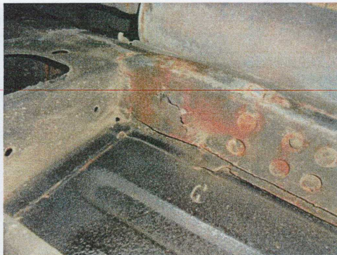
Korozja podłużnic
